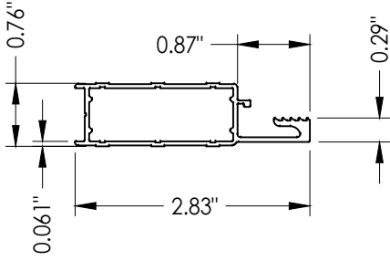
1 SCREEN DOOR FRAME
