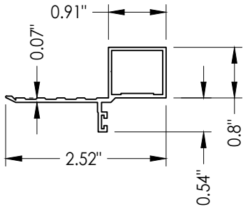
3A DOOR BUILD-OUT FRAME
